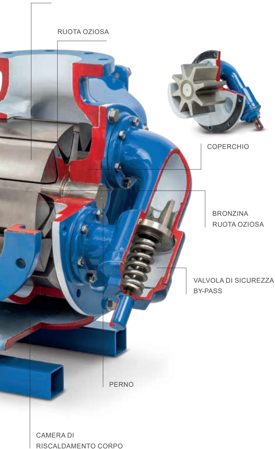
ROTORE
