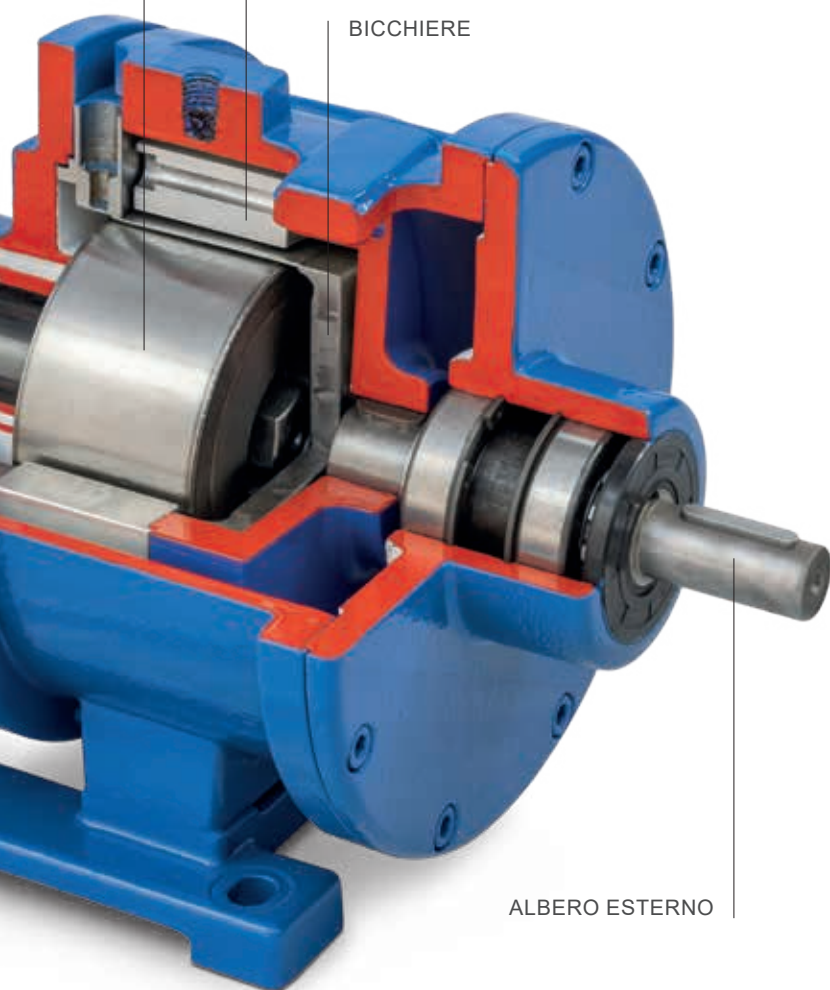
MAGNETE ESTERNO
