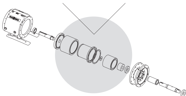
MAGNETE ESTERNO
